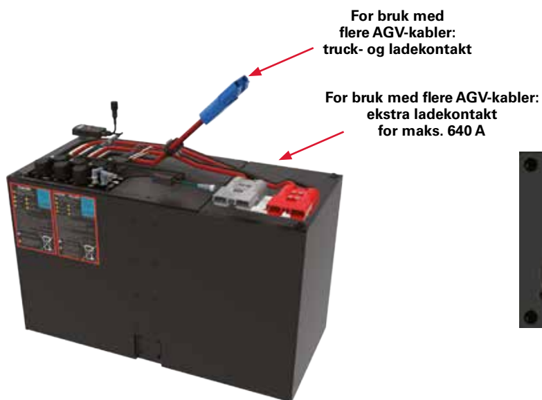
Figur 5: Bruk med flere AGV-kabler
